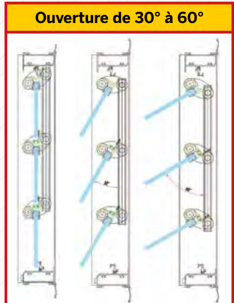
Jalousie + moustiquaire L. 600 x H. 800 Réf. GOL3110
