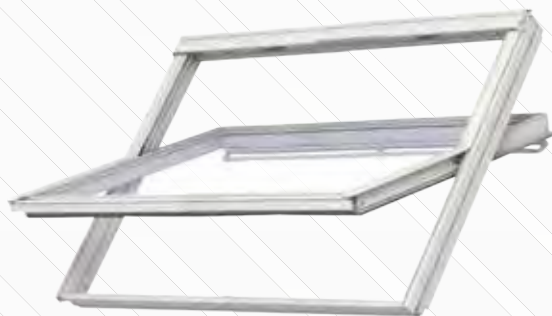
Fenêtre + raccord UK04 Velux 134 x 98 cm Velux GGL STD UK04 - Réf. VEL0002 - 130 000 F Raccord Velux EDW UK04 Gris - Réf. VEL0101 - 19 995 F
