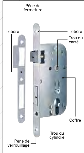
Modèle Inox Serrure - Réf. VAC0225 - 2 995 F Gache - Réf. VAC0026 - 1 735 F
