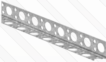
Cornière alu perforé 23,5 x 23,5 cm épaisseur 0,35 mm longueur 3 m - Réf. TPLA544
