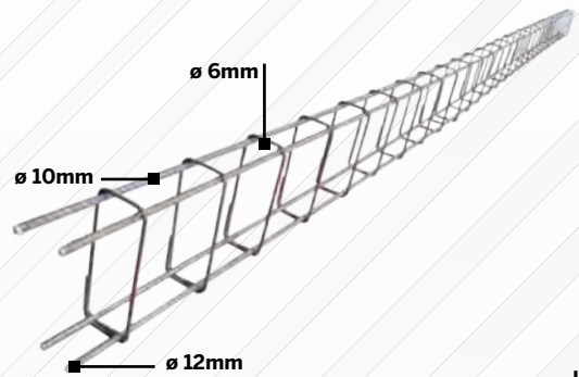
Longrine 9 x 23 x 600 cm Réf. KAFL30
