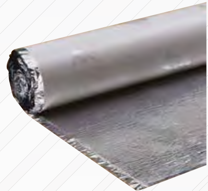
Sous-couche ALU Largeur : 1m10 Épaisseur : 2 mm Réf. SOMP903
