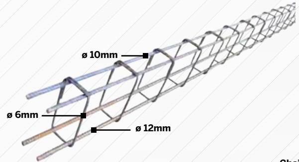
Chainage 9 x 19 x 600 cm Réf. KAFC20
