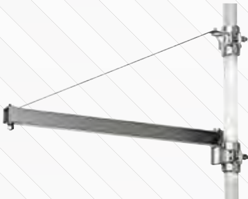
Support pour palan FARTOOLS Amovible à 180° Longueur du bras 75 à 110 cm Réf. FAR0132
